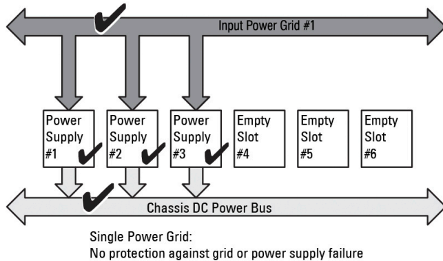
Abbildung 7. „Keine Redundanz“ bei drei Netzteileinheiten im Gehäuse
